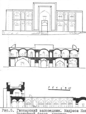
Рис.5. Гиссарский заповедник. Мадраса Нав. Восточный фасад, разрез.
