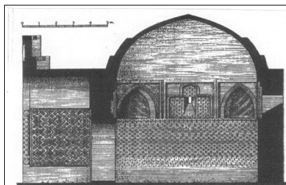
Рис. 1. Мавзолей Ходжа Нахшон (западный) Реконструкция разреза.
