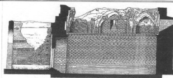
Рис. 4. Турсунзадевский район. Западный мавзолей Ходжа Нахшон, X-XI вв. Разрез (1970 г.).
