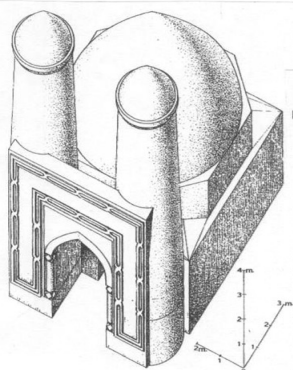
Рис. 7. Мавзолей Ходжа Нахшон, восточный, Реконструкция, Аксометрия
